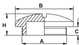
圆头
