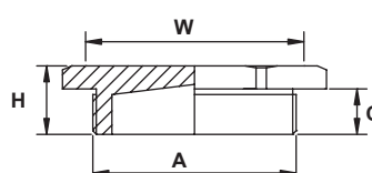
六角头
