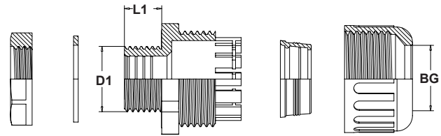
螺母 Lock Nut A 垫片 Gasket B 本体 Body C 防水圈 Seal D 迫紧头 Sealing Nut E
