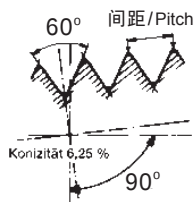
NPT型螺纹
