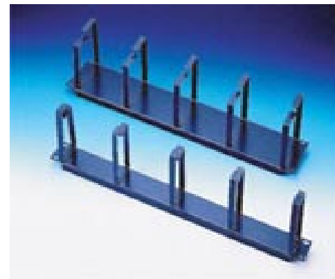
管理子系统构件：理线架
