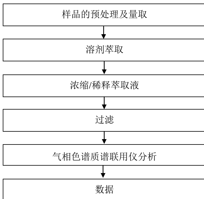
六溴环十二烷/邻苯二甲酸酯测试流程图
