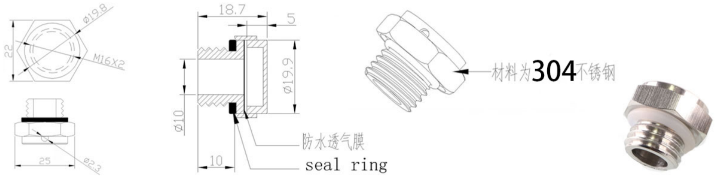
MV- M16*2.0
