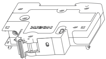
UVT欠压脱扣器 UVT Undervoltage release
