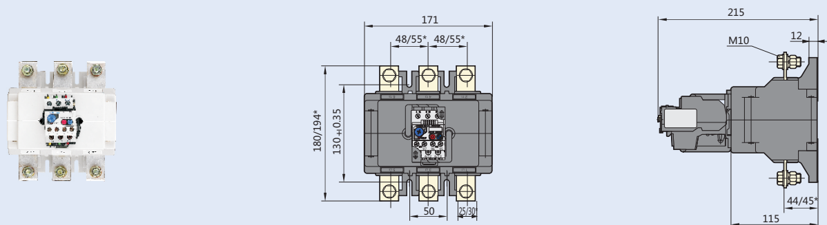
NR2-630外型及安装尺寸
