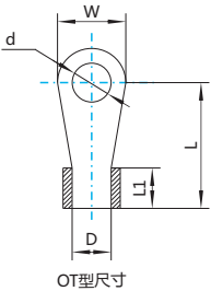
OT型尺寸
