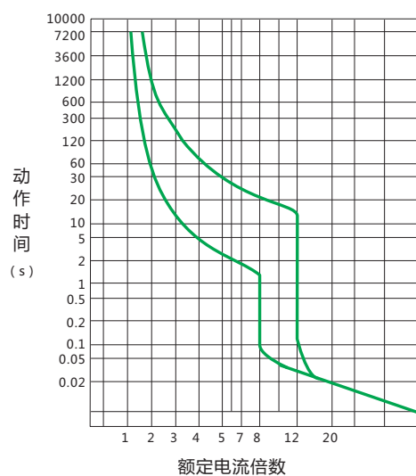
NXMLE-160
