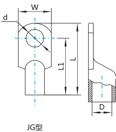
JG型
