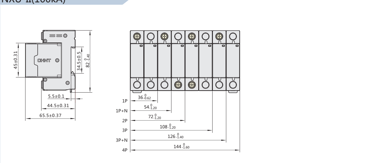
图5 不带远程信号输出接点电涌保护器外形及安装尺寸
