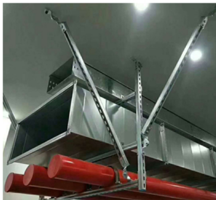
欧姆管卡固定管道应用
