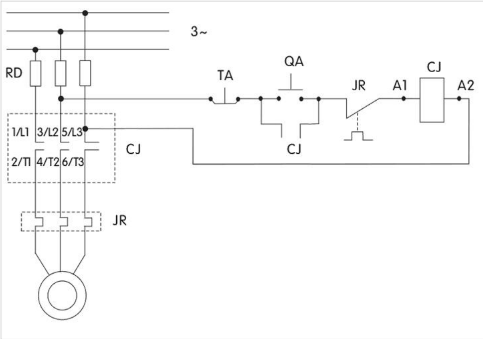
接线图 CONNECTION DIAGRAM
