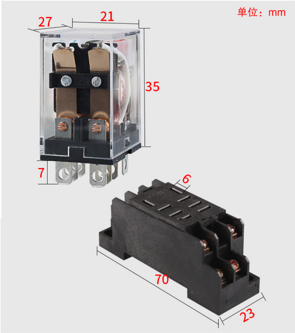
底视接线图 JQX-13F(D)
