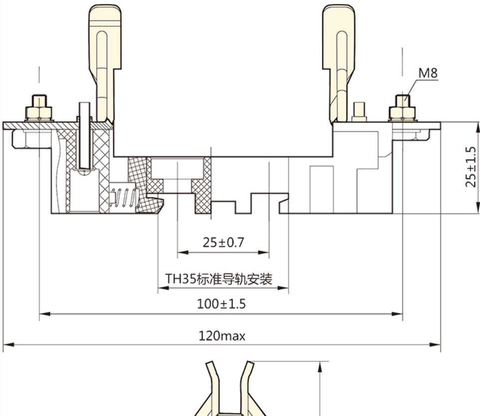
RT36-00底座
