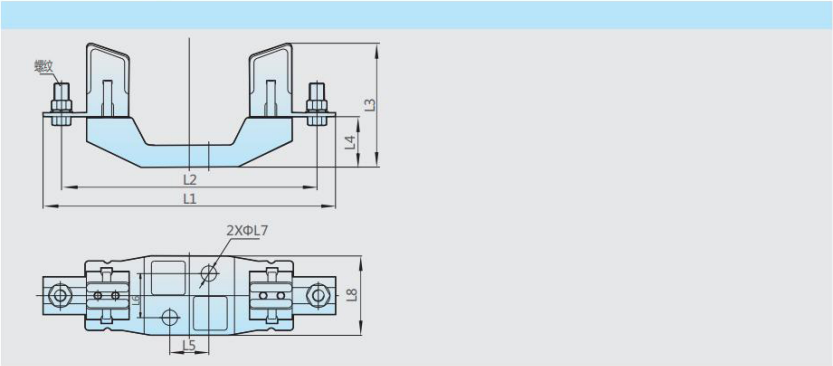
4.2 熔断器底座尺寸
