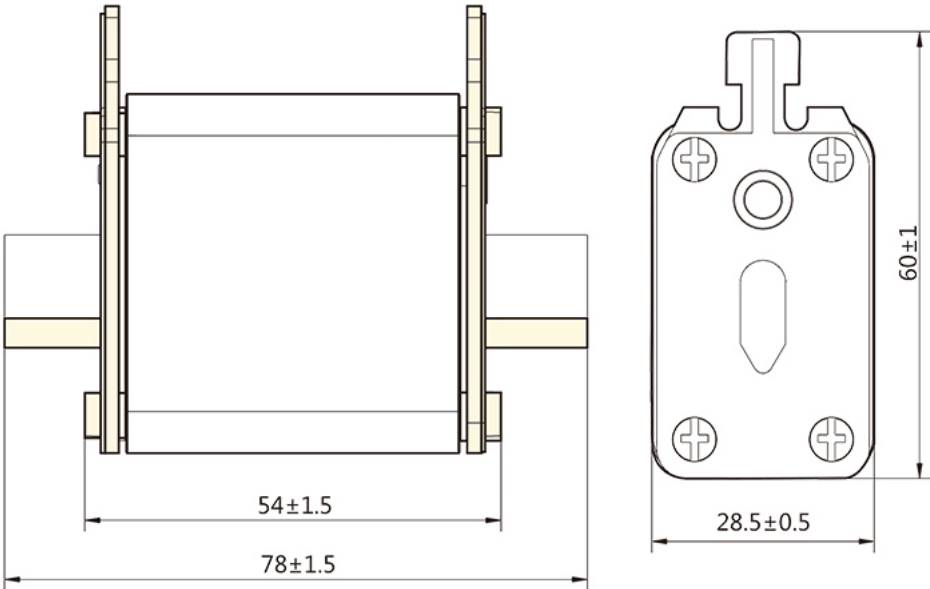
RT36-00熔断体
